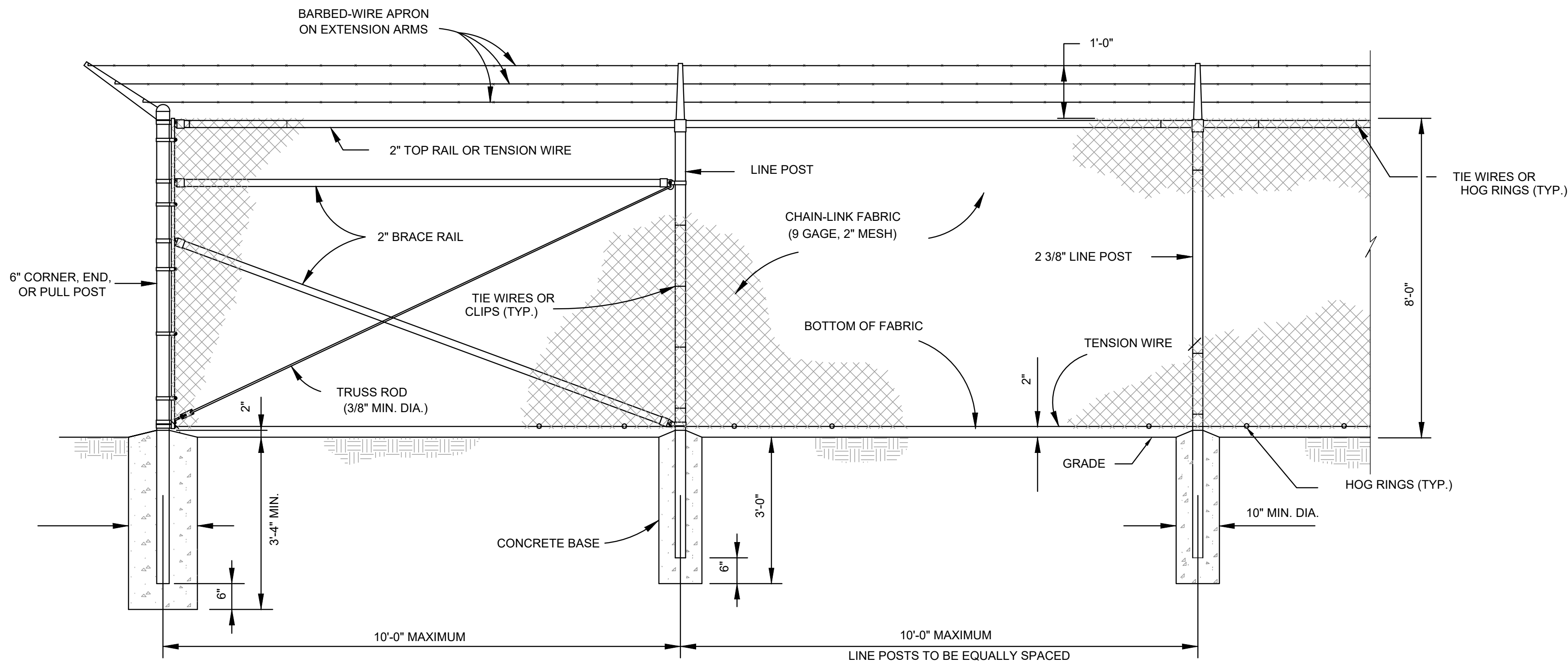
CHAIN-LINK SAFETY FENCE (H) N.T.S.
