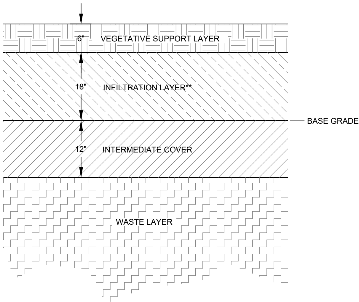
A 06 FINAL COVER DETAIL N.T.S.
